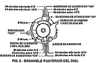
FIG. 2 - ENSAMBLE POSTERIOR DEL DIAL
