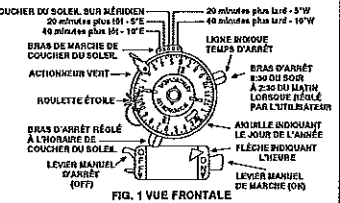
FIG. 1 VUE FRONTALE
