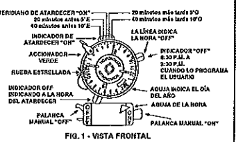
FIG. 1 - VISTA FRONTAL
