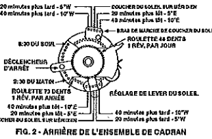
FIG. 2 - ARRIÈRE DE L'ENSEMBLE DE CADRAN
