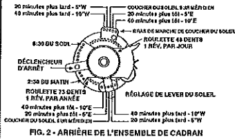
FIG. 2 - ARRIÈRE DE L'ENSEMBLE DE CADRAN
