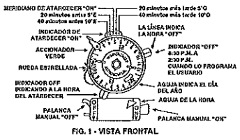
FIG. 1 - VISTA FRONTAL
