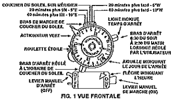
FIG. 1 - VUE FRONTALE
