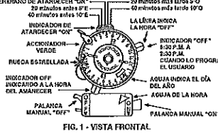
FIG. 1 - VISTA FRONTAL
