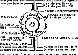
FIG. 2 - ARRIÈRE DE L'ENSEMBLE DE CADRAN
