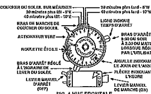
FIG. 1 VUE FRONTALE
