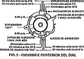
FIG. 2 - ENSAMBLE POSTERIOR DEL DIAL
